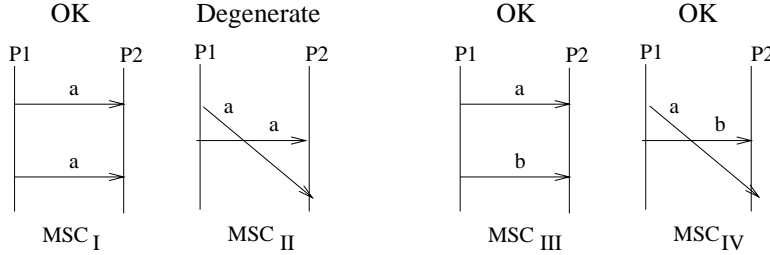
Fig. 4. Degeneracy in MSCs
