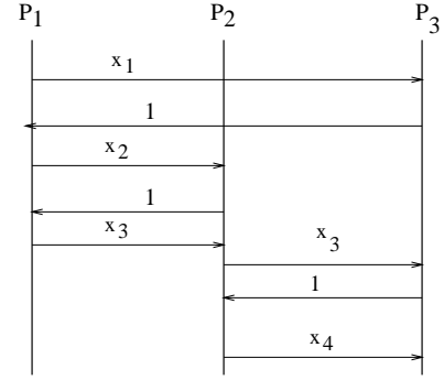
Fig. 10. The example MSC template M'
